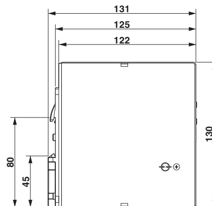
Рисунок 5 Размеры устройства (мм)
