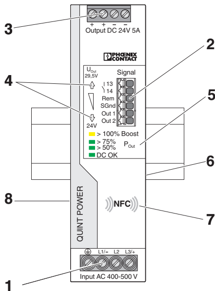
Рисунок 3 Элементы управления и индикации
