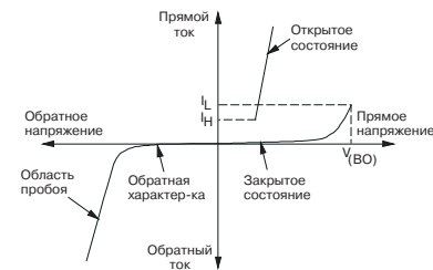
Тиристор
