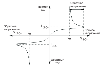
Диак (динистор)
