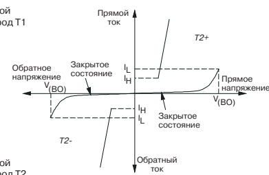
Симистор
