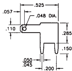
.110 TAB
