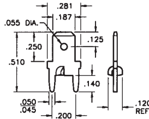
.205 TAB
