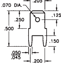
.205 TAB
