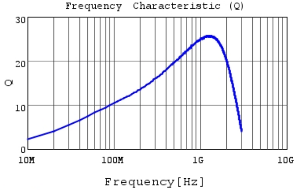
LQP03TN18NH02 Q
