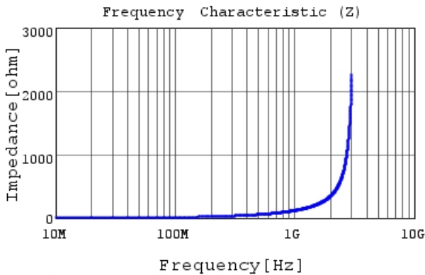
LQP03TN18NH02 |Z|
