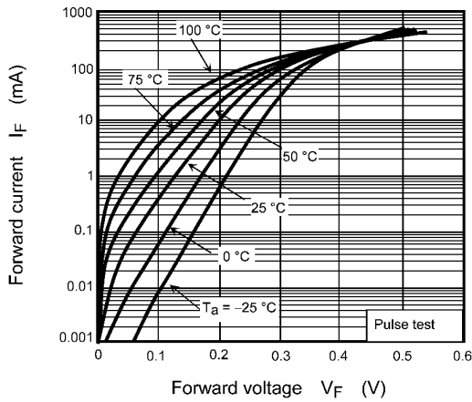
Fig. 7.2.1 I_F - V_F
