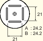
A1182 BQFP 24 × 24
