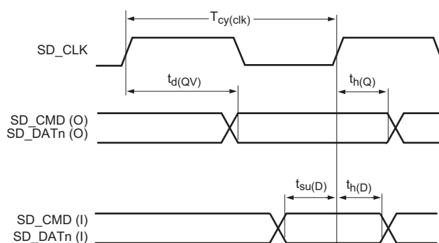
Fig 27. SD/MMC timing
