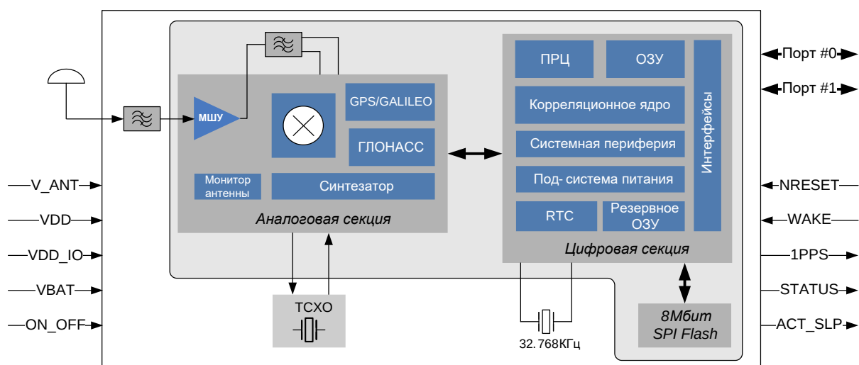
Рис. 1. Структурная схема
