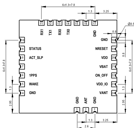
Рис. 3. Габаритный чертеж
