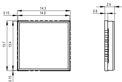
Рис. 3. Габаритный чертеж
