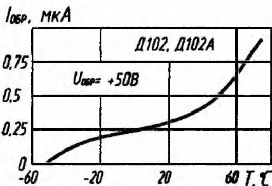
Зависимость обратного тока от температуры
