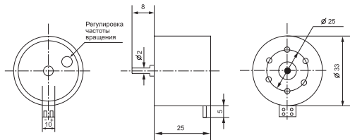
Габаритный чертёж
