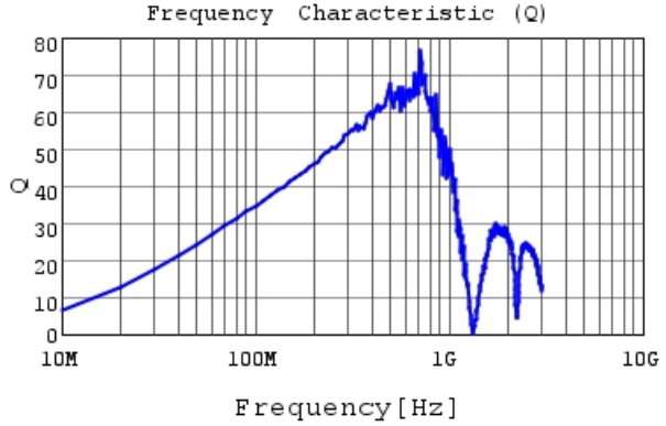
LQW18ANR27G00 Q
