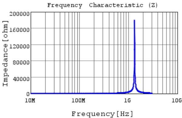
LQW18ANR27G00 |Z|
