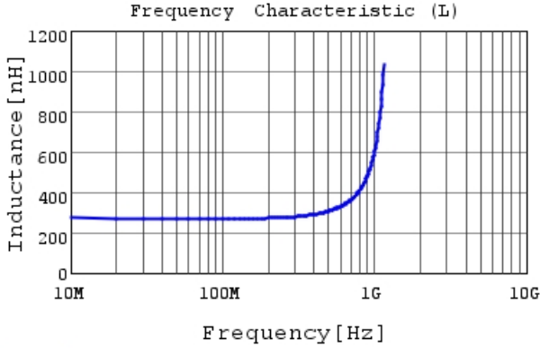
LQW18ANR27G00 L
