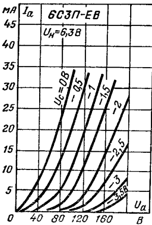
Анодные характеристики.
