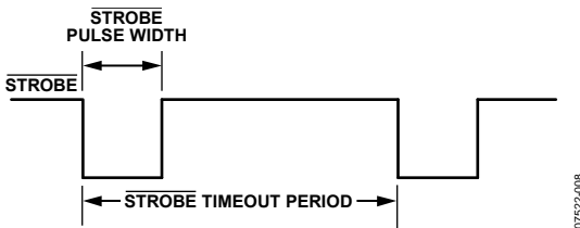
Figure 8. STROBE Parameters
