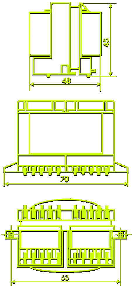
Габаритные размеры
