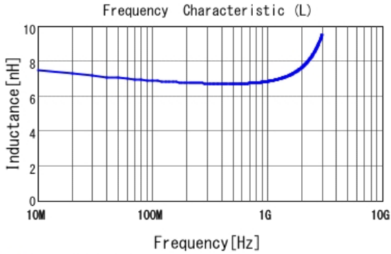
■ LQG18HN6N8J00 L
