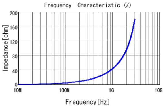
■ LQG18HN6N8J00 |Z|
