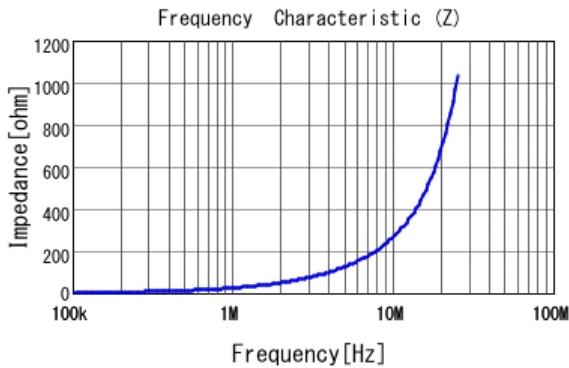
■ LQM2MPN4R7MG0 |Z|
