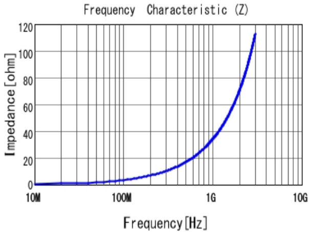
■ LQW15AN5N6D10 |Z|
