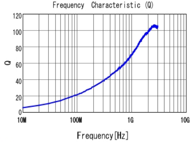
■ LQW15AN5N6D10 Q
