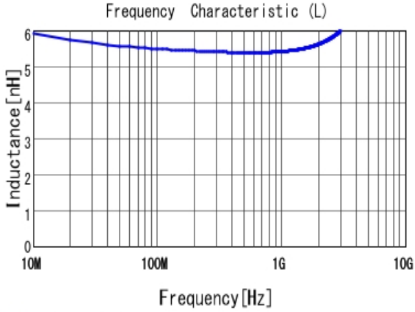
■ LQW15AN5N6D10 L
