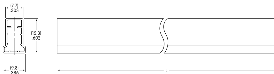
Stick-Tube Dimensions
