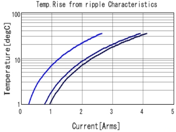
GRM316R61A475KE19 Temp. rise ■ 100kHz ■ 500kHz ■ 1MHz
