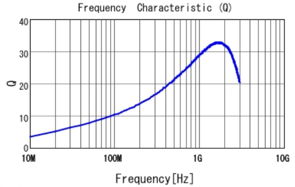
■ LQG15HS9N1J02 Q
