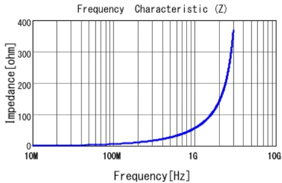
■ LQG15HS9N1J02 |Z|
