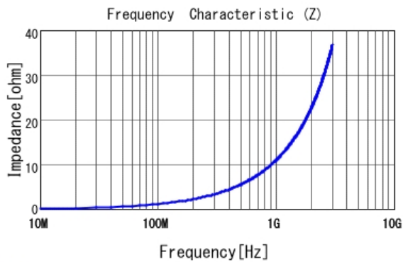
■ LQG15HN1N8S02 |Z|
