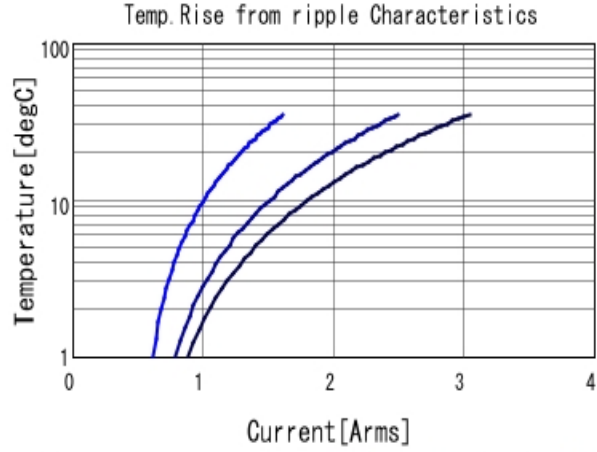
GRM188R71A474KA61 Temp. rise ■ 200kHz ■ 500kHz ■ 1MHz
