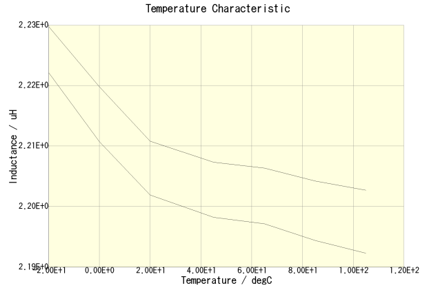
NLV32T-2R2J-PF(DC = 0A)
