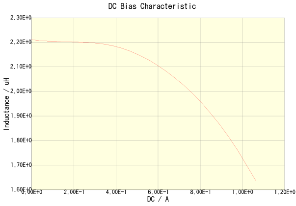
NLV32T-2R2J-PF(Amb. Temp. = 20degc)
