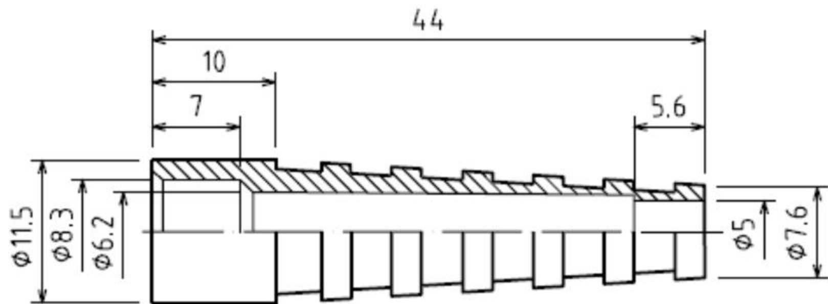
Схема BOOT58-B
