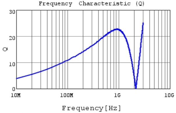
LQG15HN27NJ02 Q
