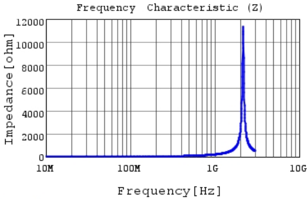
LQG15HN27NJ02 |Z|
