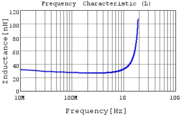
LQG15HN27NJ02 L
