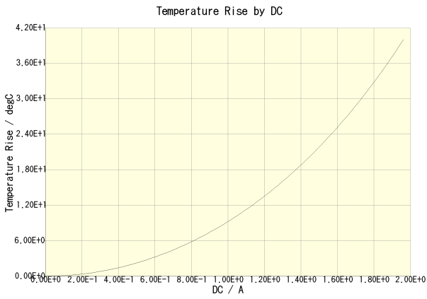
MLZ2012N1R0LT000(Amb. Temp. = 20degc)
