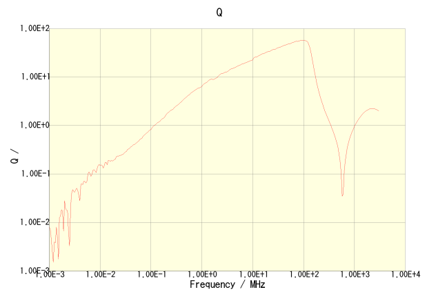
MLF2012D82NMT000
