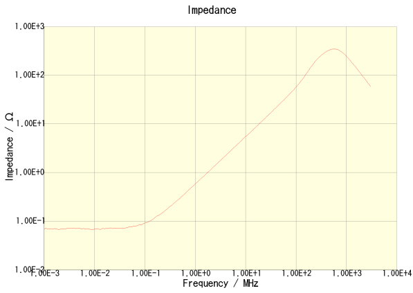
MLF2012D82NMT000
