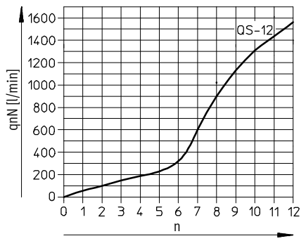
GRLA-1/2
