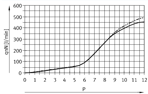
VFOH-LE-A-G14
