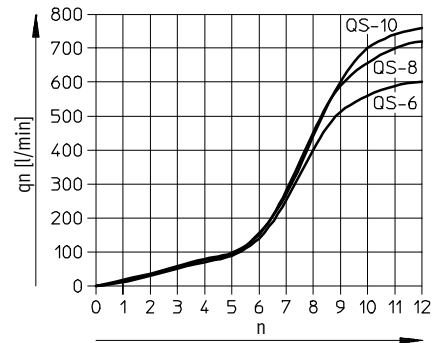
GRLA-1/8...-MF/GRLA-1/4
