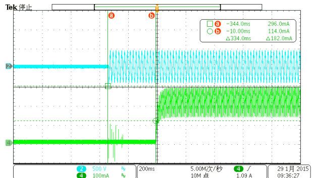
264Vac CH1: Vin CH4: I
