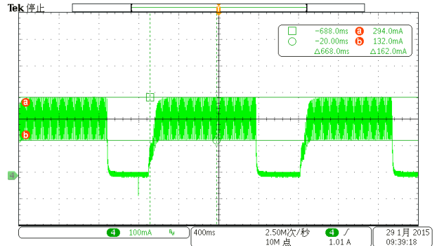
264Vac CH4: Io
