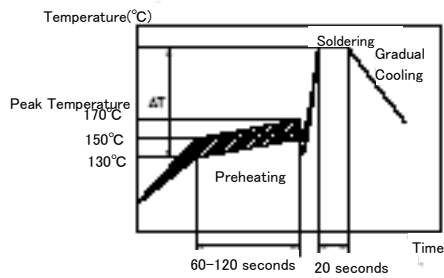
Vapor Reflow
