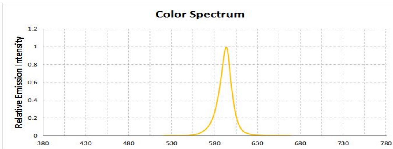
光谱图, Ta=25°C
