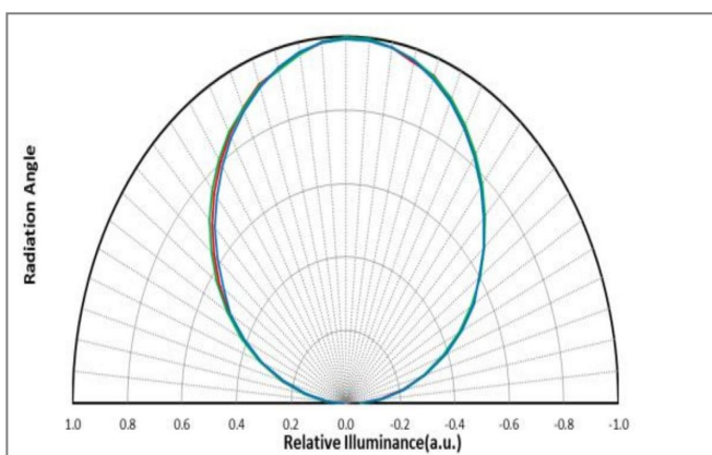
角度图, Ta=25°C
