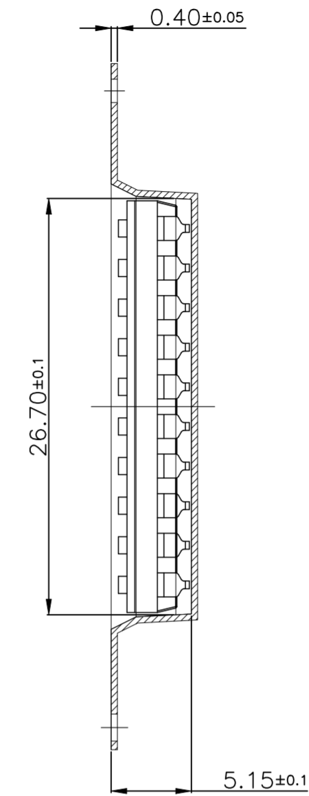
SECTION A-A
