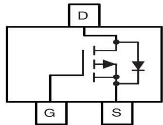
SOT-23
