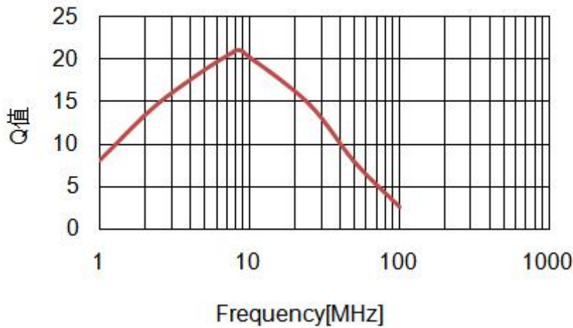
WI0603IF100KST-HF
