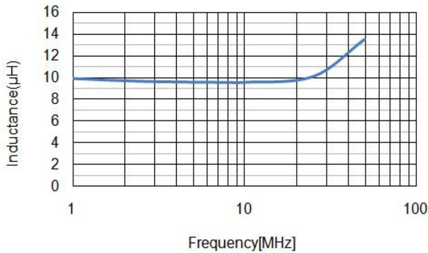
WI0603IF100KST-HF
