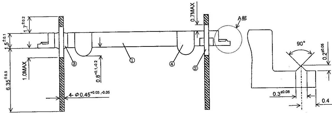
A部详图(20:1)
