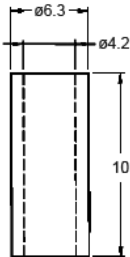
Dimensions : Millimetres
