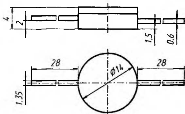
2Д2997(А-В), КД2997(А-В)
