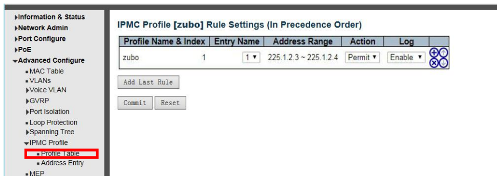
Рисунок 5-5-2 Экран настройки правила фильтрации для определенного профиля IPMS.
