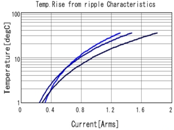
GCJ31MR72A224KA01 Temp. rise ■ 300kHz ■ 600kHz ■ 1MHz
