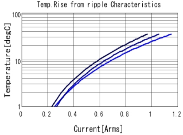
GRM1555C1H390GA01 Temp. rise ■ 500MHz ■ 700MHz ■ 1GHz
