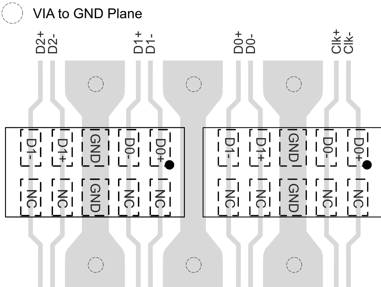
图 10-1. TPD4E05U06 Layout
