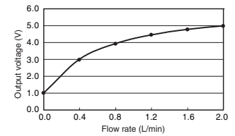
D6F-02L2-000
