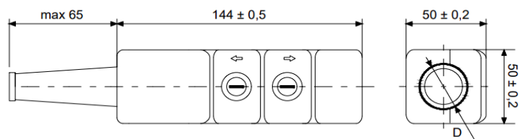
Рис.1 ПКТ-20 У2
