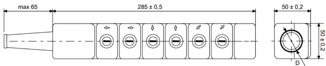
Рис3. ПКТ-60 У2
