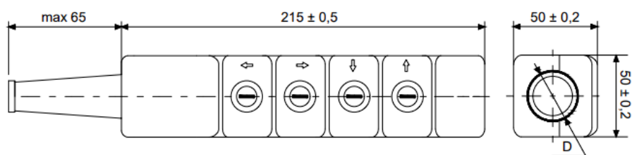
Рис.2 ПКТ-40 У2
