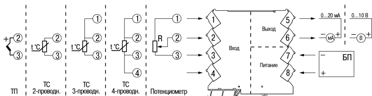
Рисунок 6.3 – Подключение прибора
