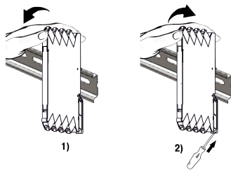
Рисунок 6.2 – Монтаж (1) и демонтаж (2) прибора
