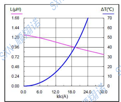
SMMS1050-1R2M
