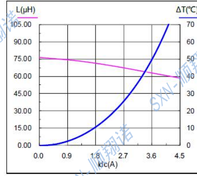
SMMS1360-820M
