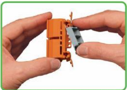
Установка на защелке углового адаптера для DIN-рейки на фиксирующий держатель.
