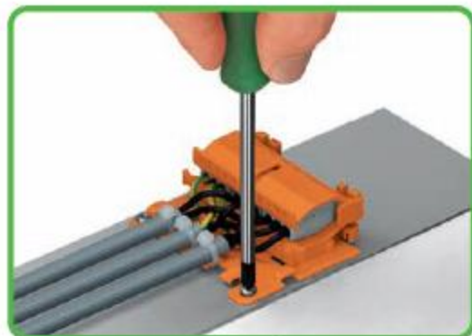
Горизонтальная установка с помощью пластины для фиксации на поверхность уровня.
