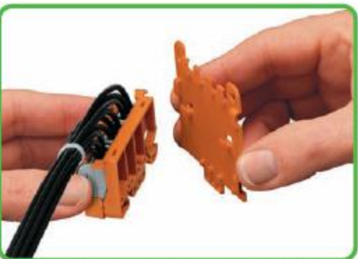
Установка пластины для фиксации на фиксирующий держатель.
