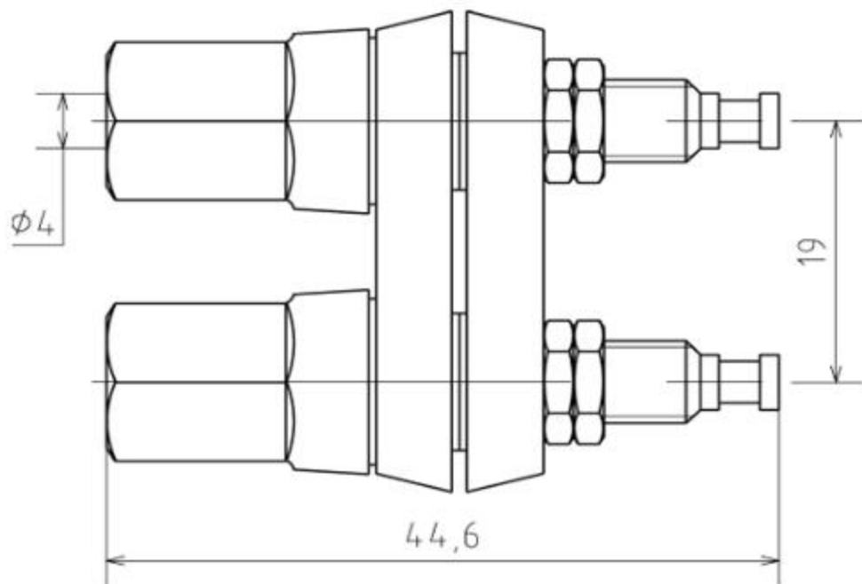
Схема BPD-1
