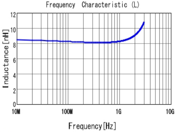
■ LQW2BAS8N2J00 L
