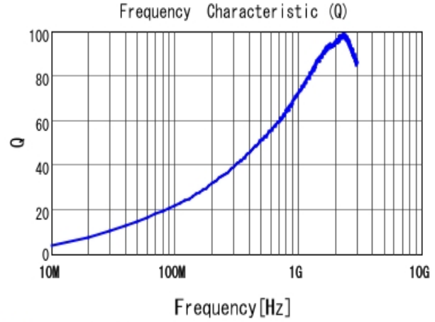
■ LQW2BAS8N2J00 Q
