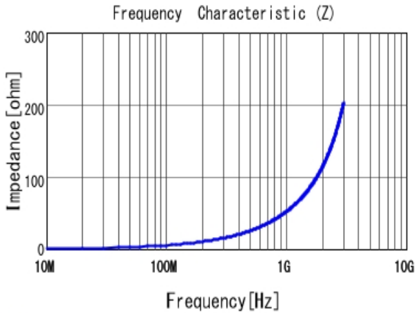
■ LQW2BAS8N2J00 |Z|
