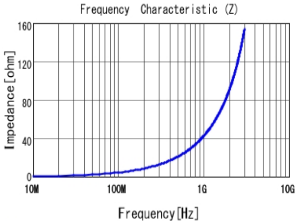
■ LQW2BAS6N8J00 |Z|
