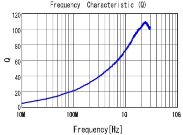
■ LQW2BAS6N8J00 Q
