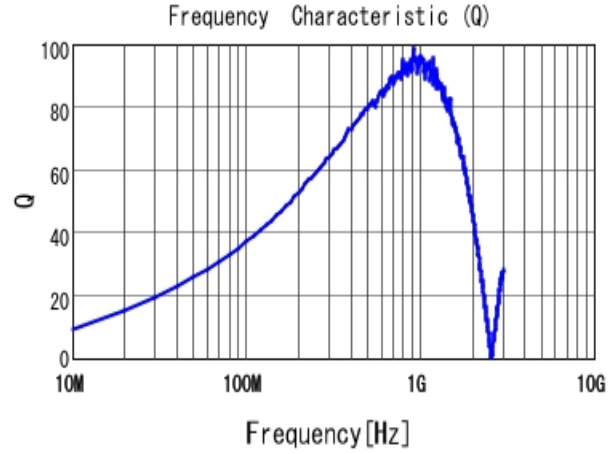
■ LQW2BAS33NJ00 Q
