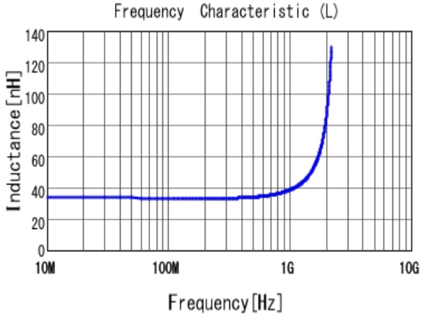
■ LQW2BAS33NJ00 L
