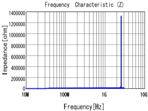
■ LQW2BAS33NJ00 |Z|
